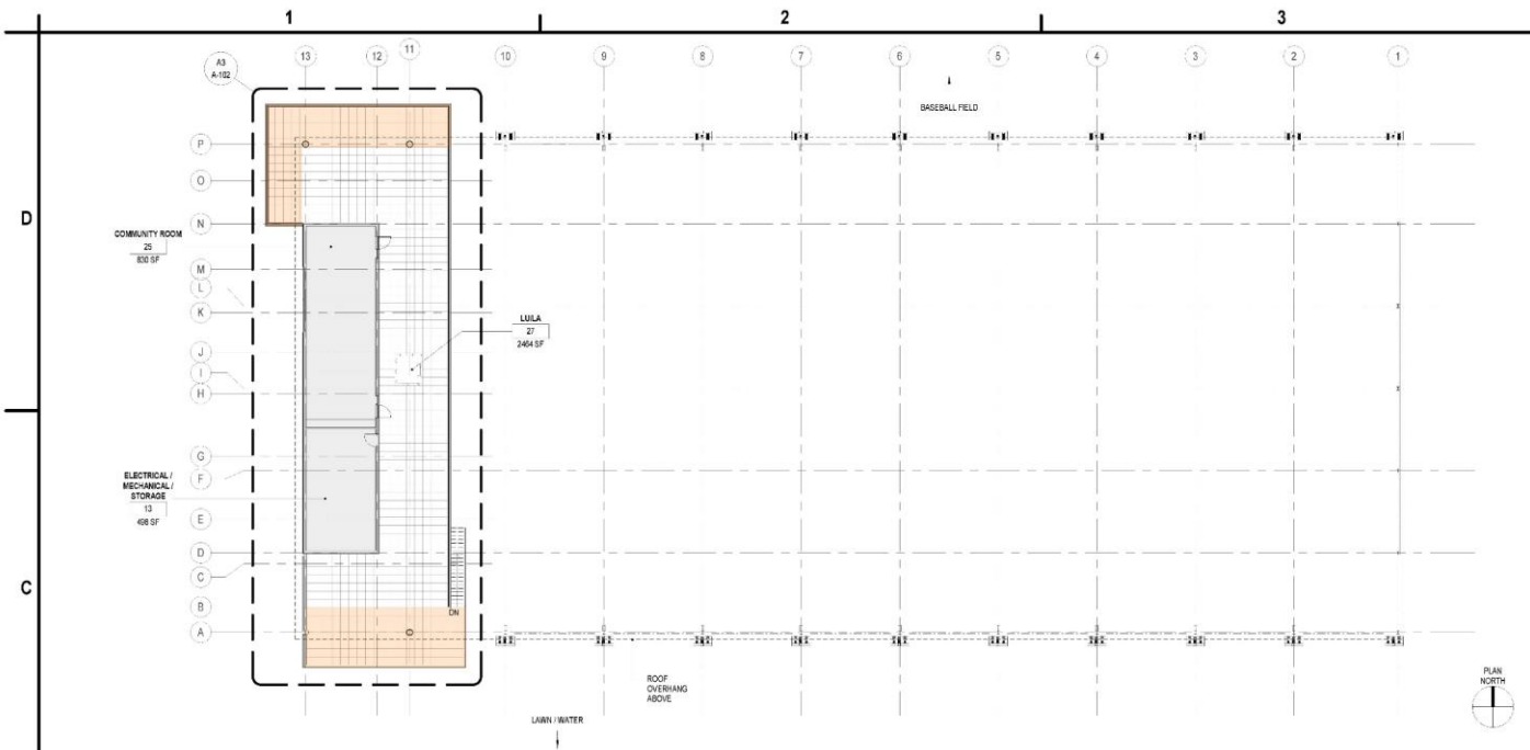
C1 MEZZANINE LEVEL SCALE: 1/16" = 1'-0"
