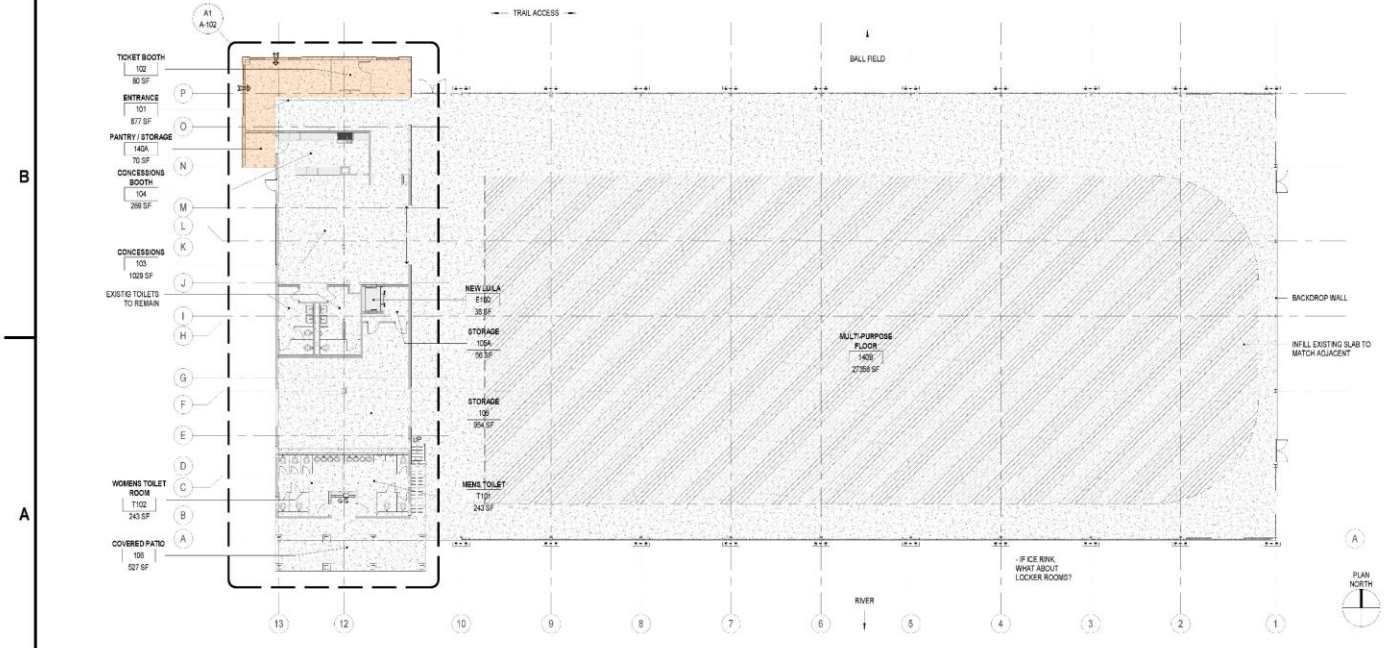
A1 MAIN LEVEL SCALE: 1/16" = 1'-0"
